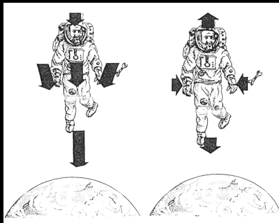
slapové působení: v soustavě Země...
