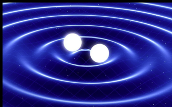
system dvou neutronových hvězd obíhajících velmi blízko sebe
