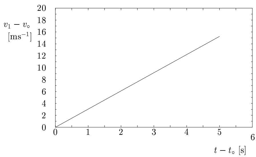
Obr. 3: Graf závislosti velikosti rychlosti podstavec – podložka na čase
