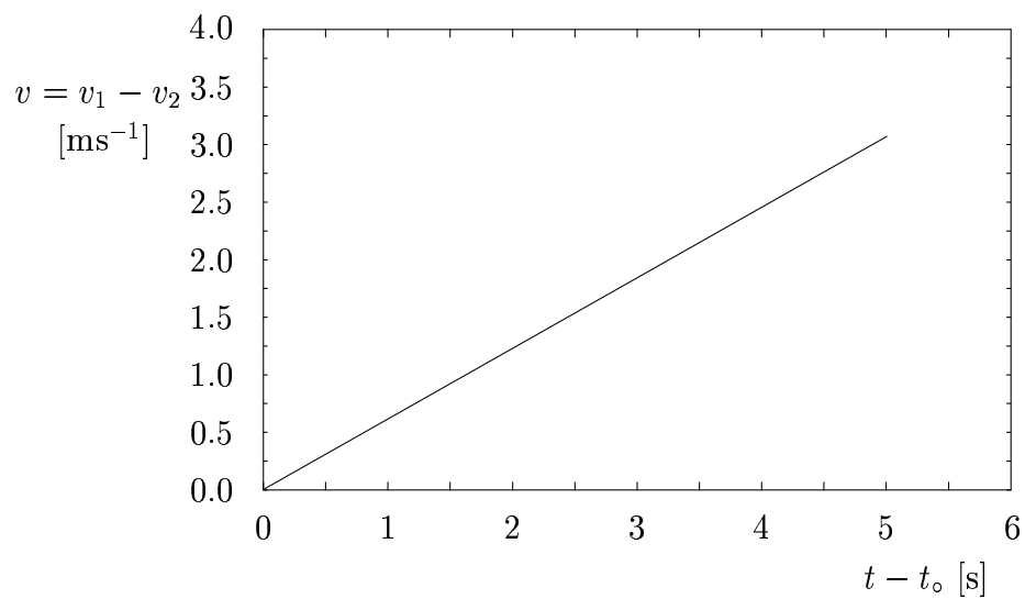
Obr. 5: Graf závislosti velikosti rychlosti hranol – podstavec na čase
