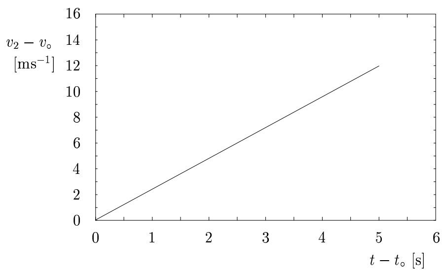
Obr. 4: Graf závislosti velikosti rychlosti hranol – podložka na čase
