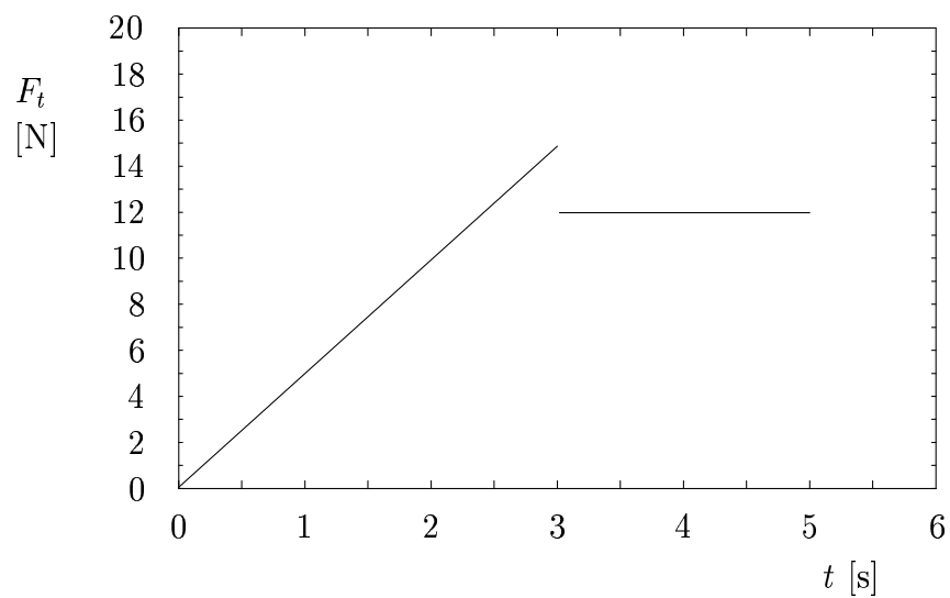
Obr. 1: Graf závislosti velikosti třecí síly na čase
