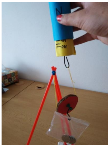
Obr. 3. Kladka volná.
