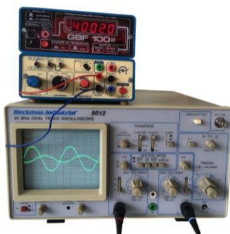
Obr. 2. Generátor napětí GBF 100 a dvoukanálový osciloskop.
