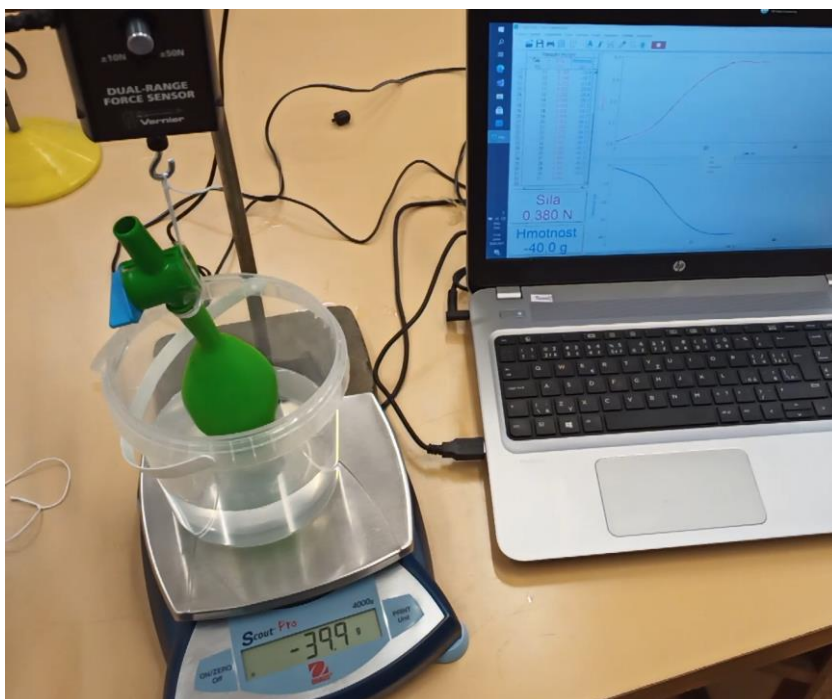
Obr. 1. Uspořádání experimentu s vyfukováním balónku
